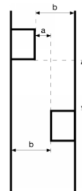
Figur 4.33 Forsætning med indsnævring, bestemmende mål
